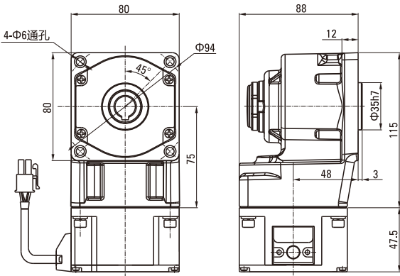
输出轴结构
